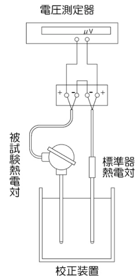
図-10 偏差法
