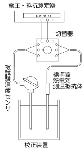
図-9 比較試験
