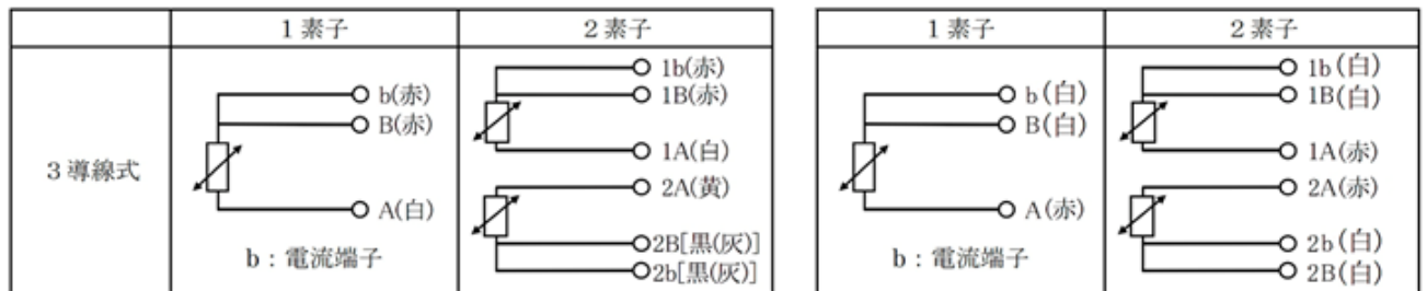
図-4 結線方式
