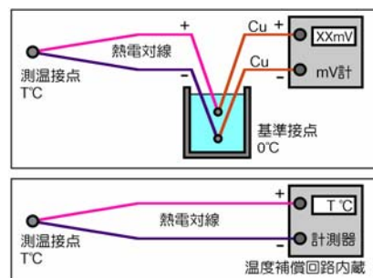
図-2 熱電対の回路
